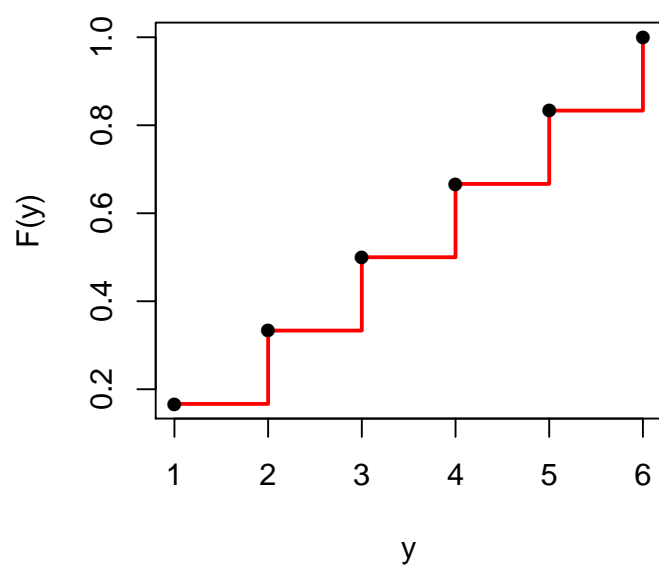
Figura 6.19: La densidad y distribución de probabilidades para un dado de seis caras
