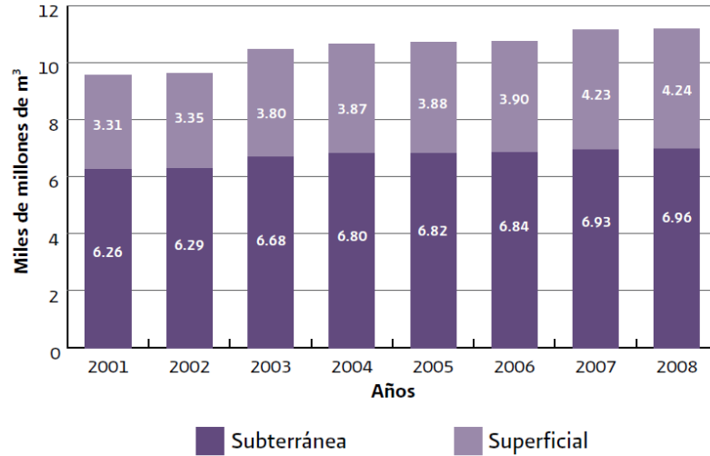
Figura 23. Concesiones de agua para consumo humano. Fuente: CONAGUA, 2010
