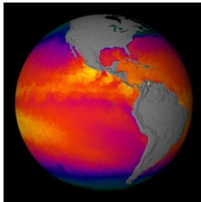
Figura 9. Gradiente de temperatura del agua en los océanos
