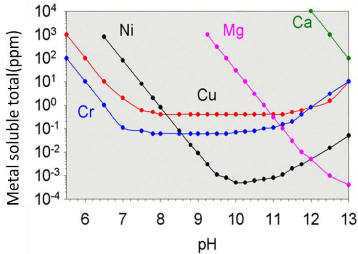
Figura 21. La solubilidad total de varios metales en agua como función del pH (Dyer et al., 1998)
