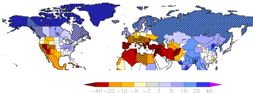
Figura 13. Cambio proyectado en la escorrentía del agua en el 2050 (Milly et al. , 2005)
