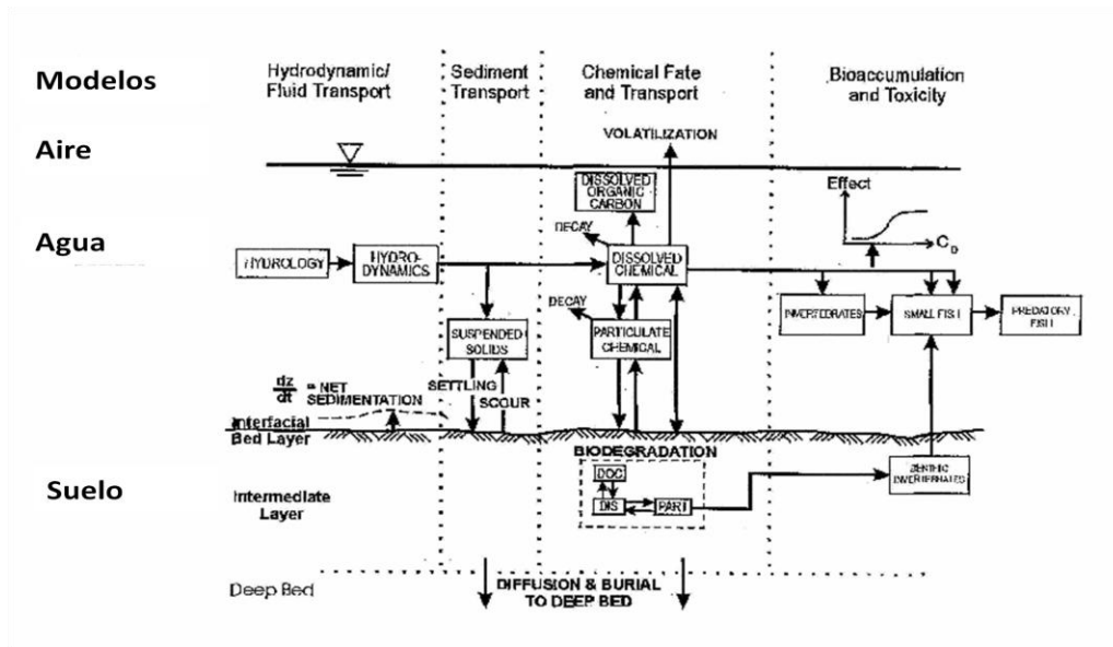
Figura 22. Estructura modelo para el transporte químico y destino en un sistema acuático (Paquin et al., 2003)
