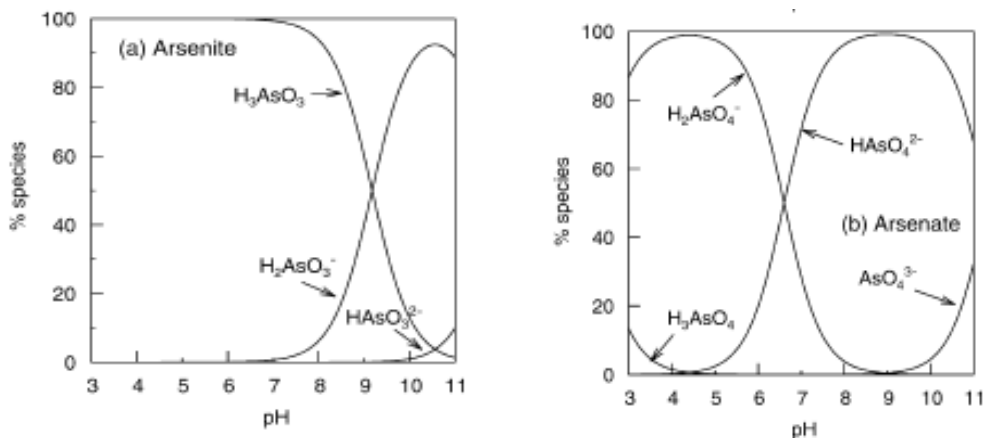
Figura 15. Especiación arsenito/arsenato como una función del pH (fuerza ionica 0.01 M)
