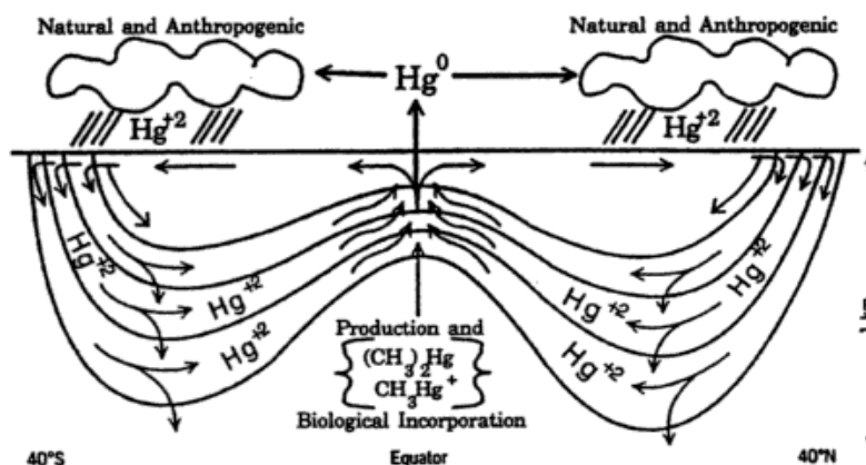
Figura 20. Representación esquemática de los patrones de circulación y transporte del mercurio, para las capas de mezcla y termoclina en el Océano Pacífico
