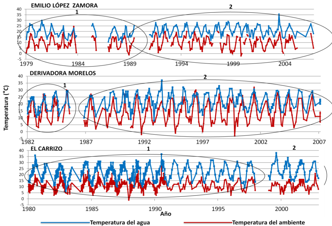
Figura 45. Gráficas Emilio López, Derivadora Morelos y El Carrizo
