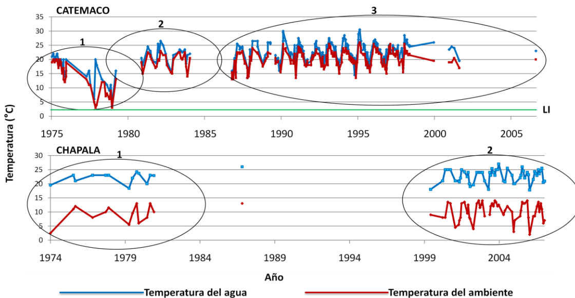
Figura 44. Gráficas de referencia de Catemaco y Chapala
