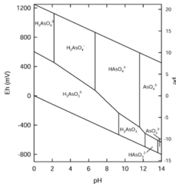
Figura 14. Diagrama pH-Eh para especies acuáticas de arsénico en el sistema As-O 2 -H 2 O a 25°C y 1 atm de presión barométrica
