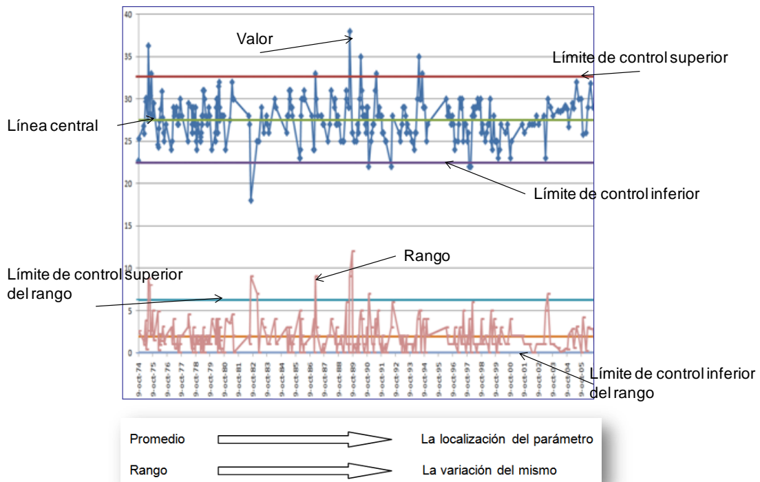
Figura 33. Gráfica de control de promedios y rangos móviles
