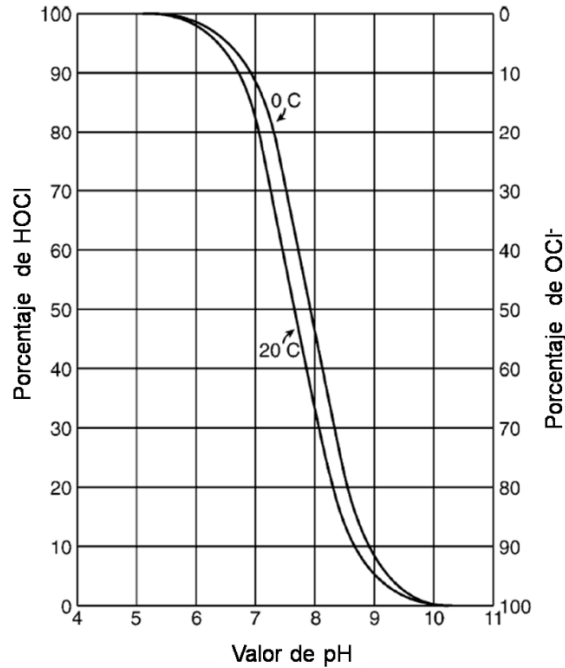
Figura 27. Distribución del ácido hipocloroso y los iones de hipoclorito en agua a distintos valores de pH y temperatura (Morris, 1982)
