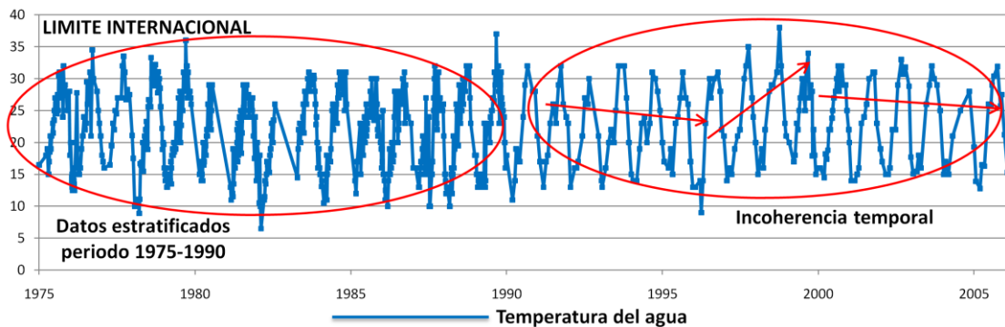
Figura 43. Estratificación de datos en el sitio Límite Internacional
