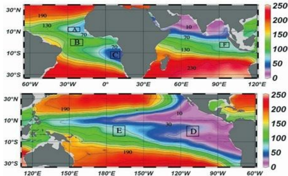
Figura 30. Promedio climatológico de las concentraciones de oxígeno disuelto (Stramma et al. , 2008)
