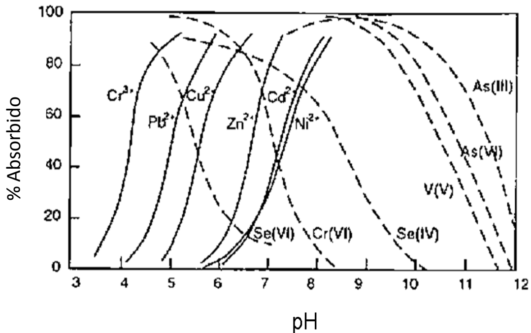
Figura 1. Adsorción de metales de acuerdo al pH
