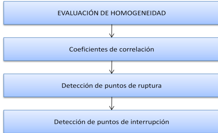
Figura 35. Proceso de evaluación de homogeneidad de la serie de datos
