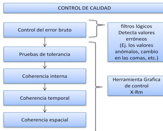
Figura 34. Proceso de control de calidad de los datos
