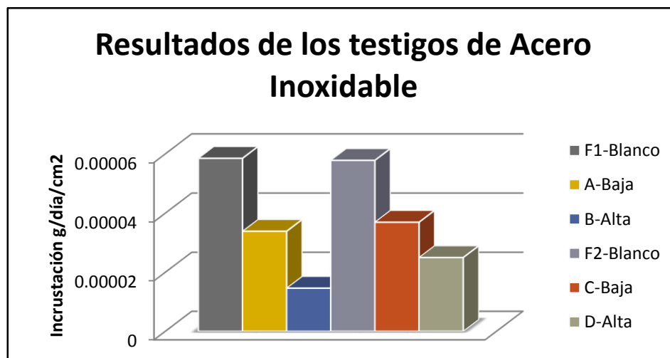
Gráfica 12. Resultados de los testigos de incrustación fabricados con acero inoxidable.
