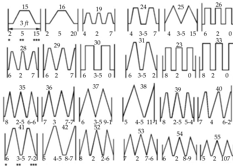
Figura 2. Modelos de los vertedores de cresta larga reportados por Hay y Taylor (1970).
