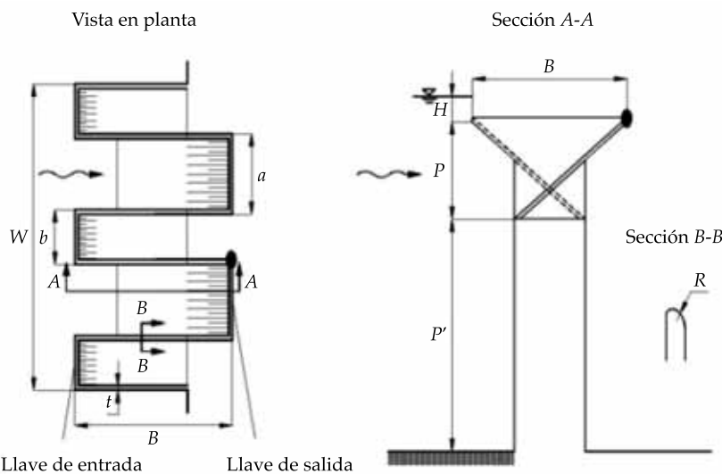
Figura 3. Planta y perfil del vertedor "tecla de piano" (Ribeiro et al., 2012).
