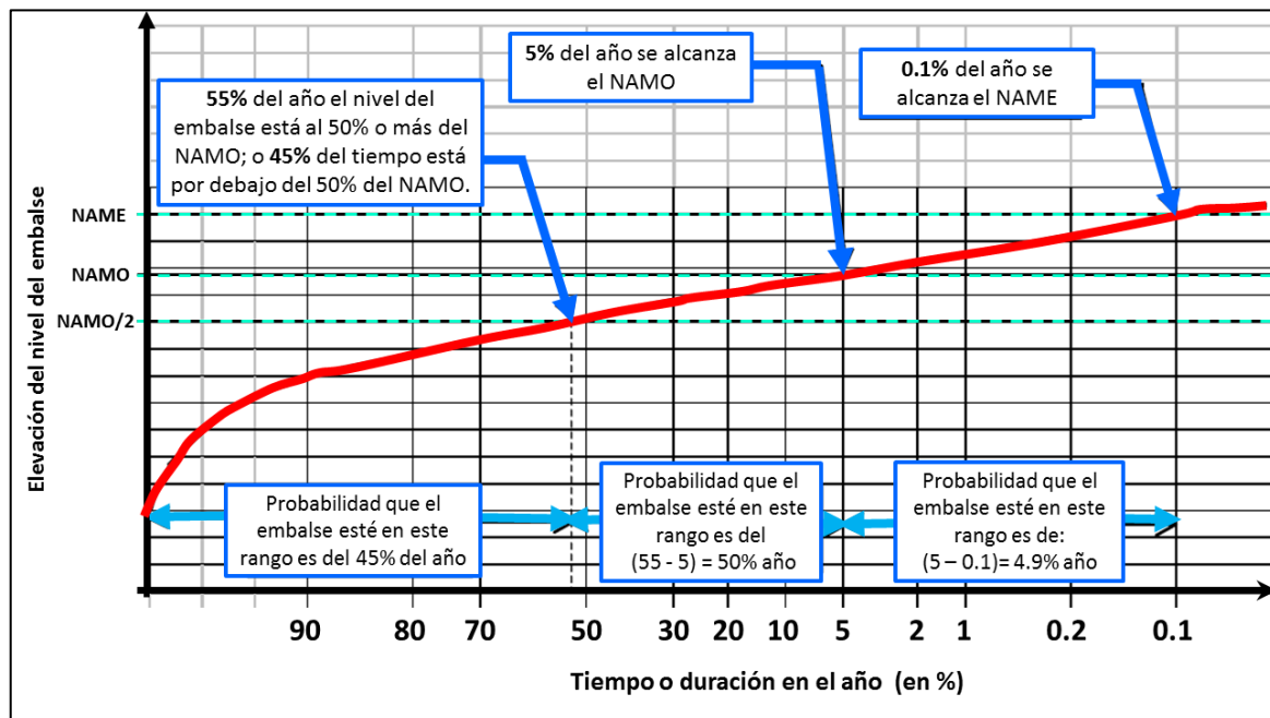
Figura 1.7 Se consideran distintos niveles del embalse, incluyendo el caso de desbordamiento que permite modelar los cambios de pendientes y pérdida de suelo de la cortina.
