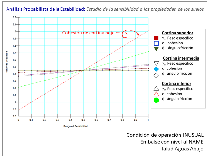
Figura 1.11 Análisis de sensibilidad y estabilidad del talud seco con el embalse lleno al NAME.
