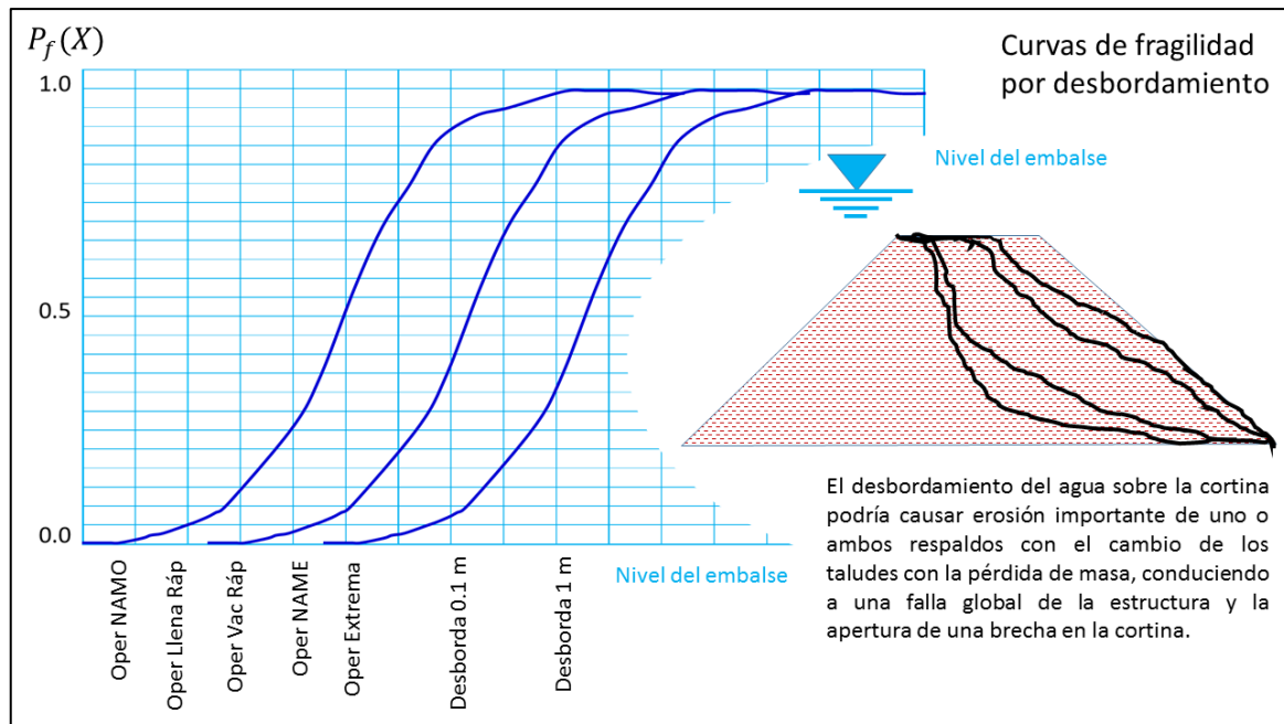
Figura 1.28 Curvas de fragilidad por la sensibilidad de la cortina en condiciones de desbordamiento.
