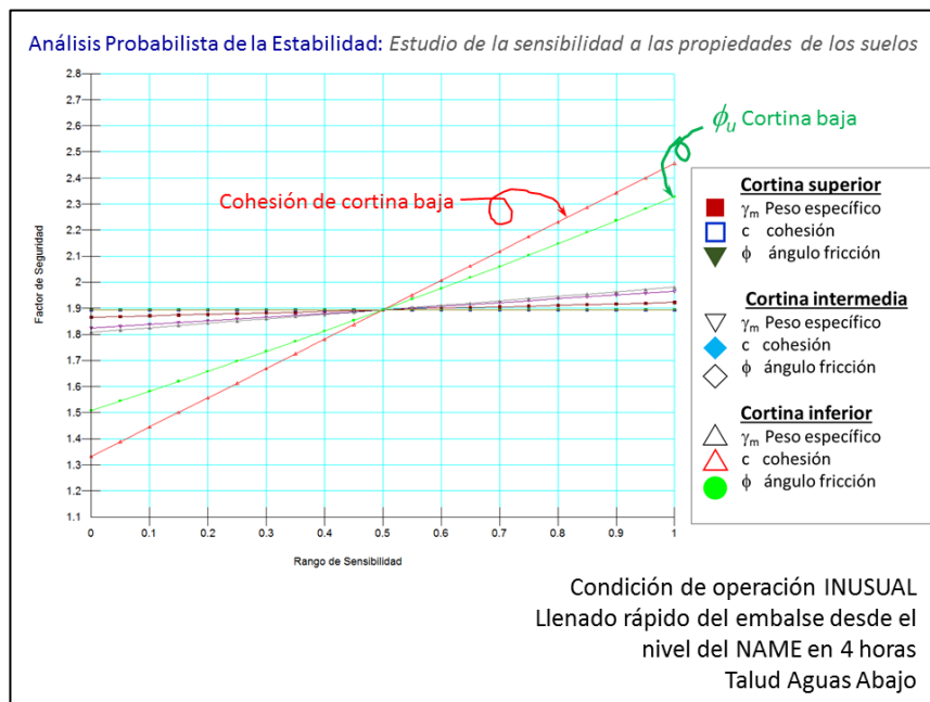
Figura 1.15 Análisis de sensibilidad y estabilidad del talud seco durante un llenado rápido.
