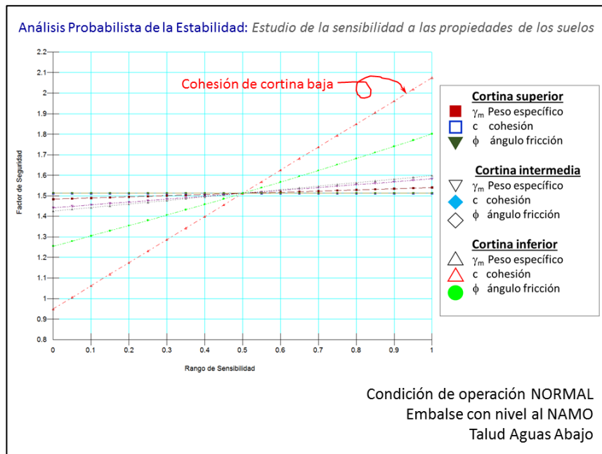
Figura 1.9 Análisis de sensibilidad y estabilidad del talud seco con el embalse al NAMO.
