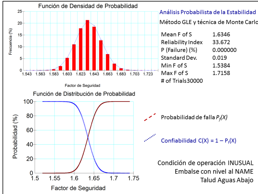
Figura 1.21 Análisis probabilista de estabilidad del talud seco con el embalse lleno al NAME.
