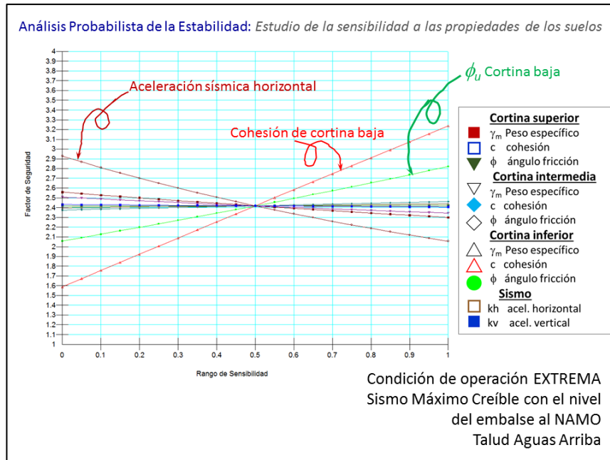
Figura 1.16 Análisis de sensibilidad y del talud mojado durante el sismo y nivel del NAMO.
