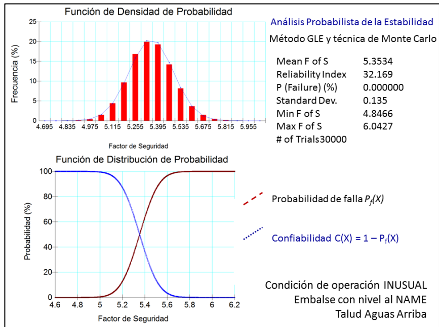
Figura 1.20 Análisis probabilista de estabilidad del talud mojado con el embalse lleno al NAME.
