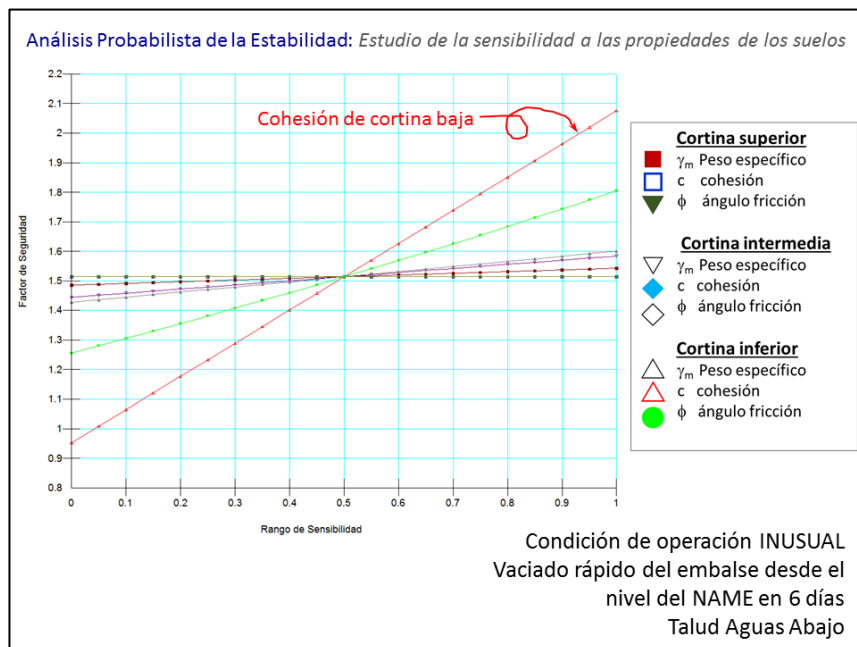
Figura 1.13 Análisis de sensibilidad y estabilidad del talud seco durante un vaciado rápido.
