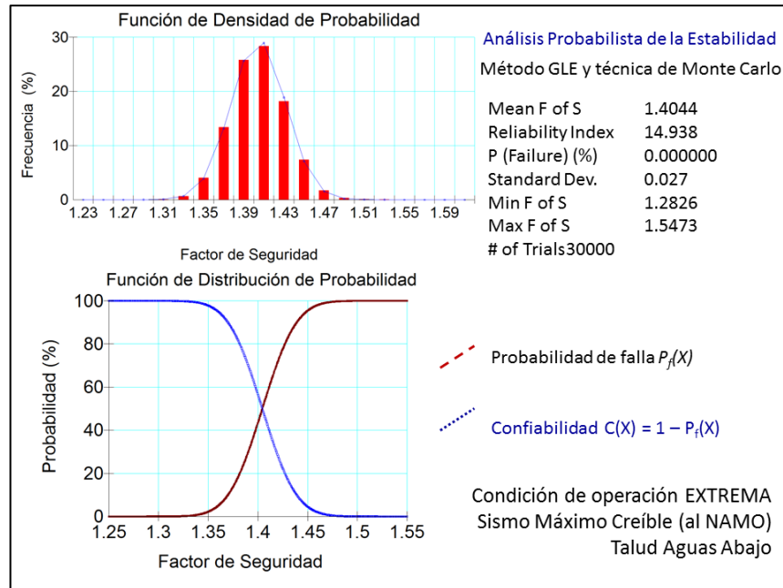
Figura 1.27 Análisis probabilista del talud seco durante el sismo con embalse al nivel del NAMO.
