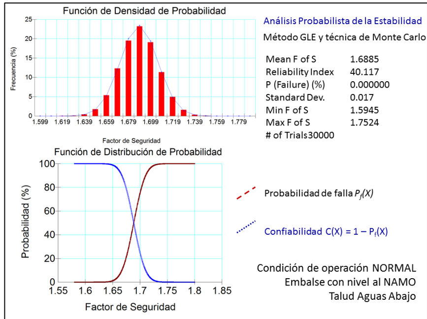
Figura 1.19 Análisis probabilista de estabilidad del talud seco con el embalse al nivel del NAMO.
