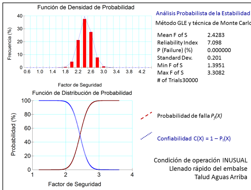
Figura 1.24 Análisis probabilista de estabilidad del talud mojado durante un llenado rápido.
