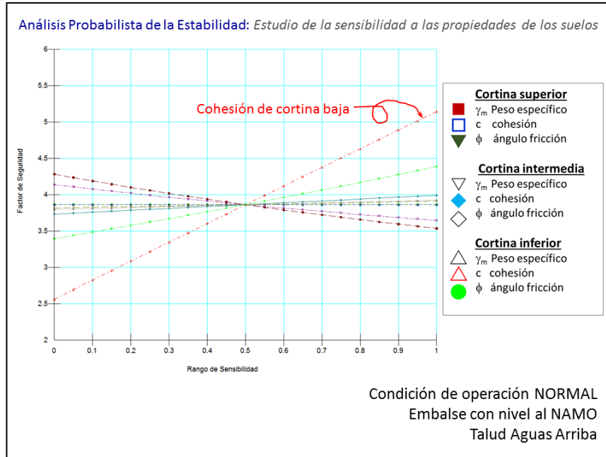
Figura 1.8 Análisis de sensibilidad y estabilidad del talud mojado con el embalse al NAMO.
