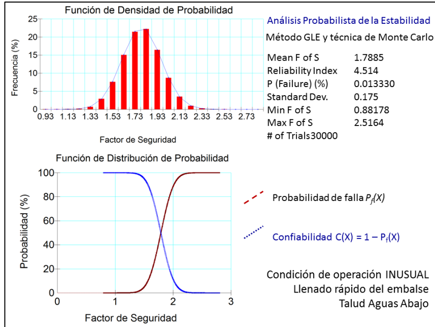
Figura 1.25 Análisis probabilista de estabilidad del talud seco durante un llenado rápido.
