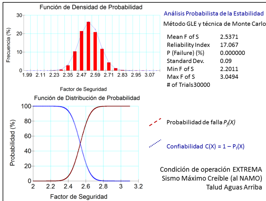
Figura 1.26 Análisis probabilista del talud mojado durante el sismo con embalse al nivel del NAMO.
