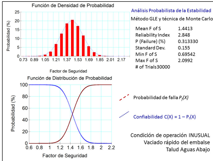
Figura 1.23 Análisis probabilista de estabilidad del talud seco durante un vaciado rápido.
