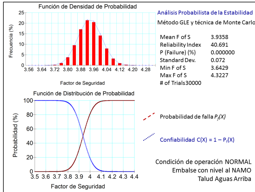
Figura 1.18 Análisis probabilista de estabilidad del talud mojado con el embalse al nivel del NAMO.
