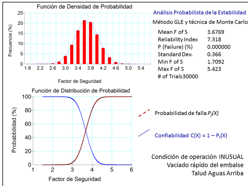
Figura 1.22 Análisis probabilista de estabilidad del talud mojado durante un vaciado rápido.
