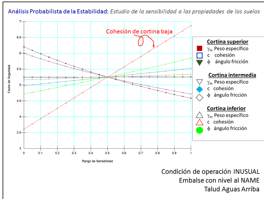
Figura 1.10 Análisis de sensibilidad y estabilidad del talud mojado con el embalse lleno al NAME.
