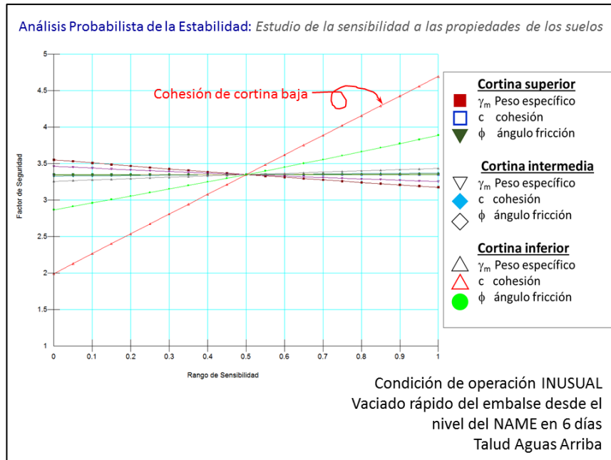
Figura 1.12 Análisis de sensibilidad y estabilidad del talud mojado durante un vaciado rápido.
