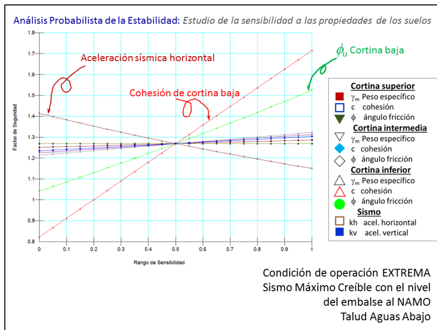
Figura 1.17 Análisis de sensibilidad y del talud seco durante el sismo y nivel del NAMO.
