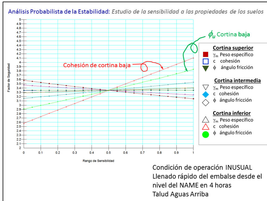
Figura 1.14 Análisis de sensibilidad y estabilidad del talud mojado durante un llenado rápido.
