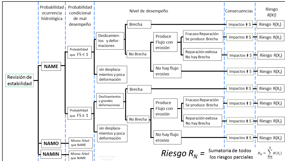
Figura 1.6 Árbol de eventos de la presa por deslizamiento.
