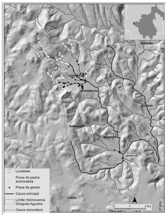
Figura 2. Ubicación de la microcuenca Choguita y de las obras de conservación de suelo.
