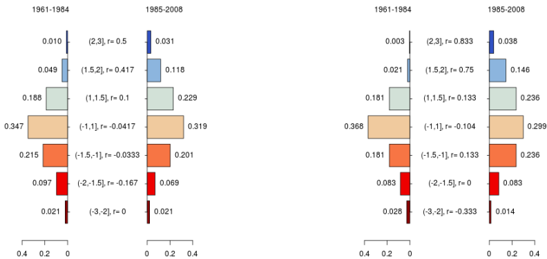
Figura 6. Fracción de cambio de SPI-6 (izquierda) y SPI-12 (derecha) promediado para toda la cuenca, comparando los periodos antiguos (1961-1984) y reciente (1985-2008)
