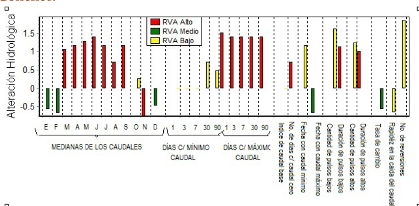
Figura 17 Alteración de los caudales ecológicos de la cuenca alta en el río Conchos.
