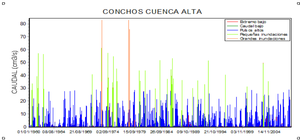
Figura 16 Componentes del caudal ecológico para la parte alta del río Conchos.
