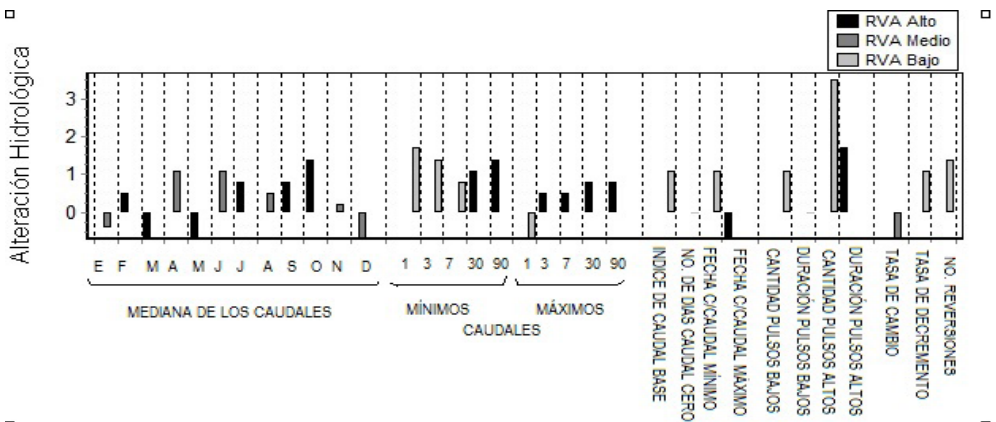
Figura 20 Alteración de los caudales ecológicos de la cuenca baja en el río Conchos.
