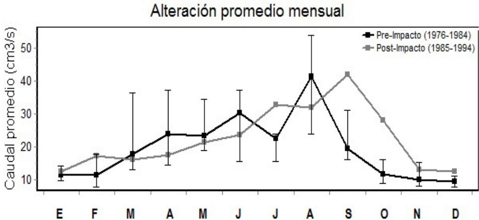
Figura 18 Caudales promedio mensual en la cuenca baja del río Conchos y en la presa La Boquilla para los periodos anterior y posterior después de la construcción de la presa.
