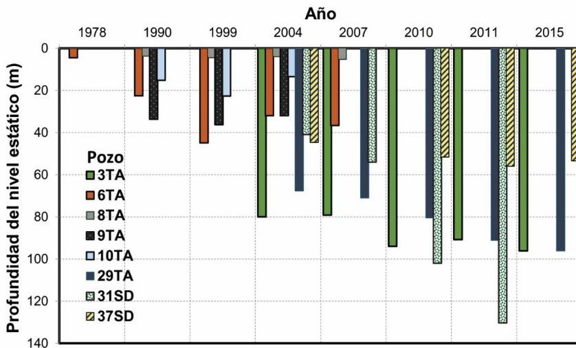
Figura 2. El gráfico presenta abatimiento de pozos muestreados dos años o más en acuíferos TA y SD.
