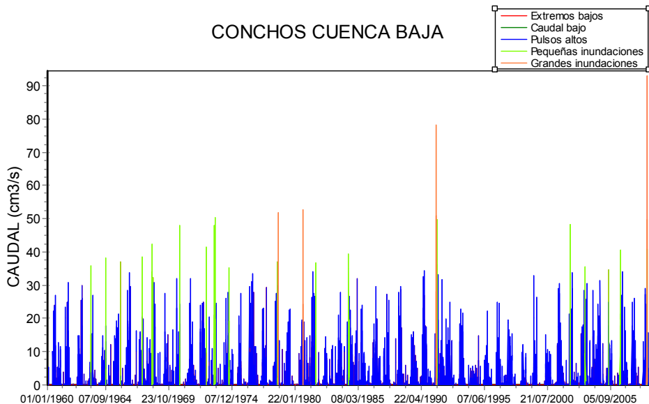
Figura 19 Componentes del Caudal Ecológico o Ambiental (EFC)
