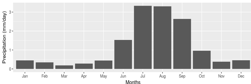
Figura 4. Ciclo medio anual de precipitación (mm/día) en la cuenca del río Conchos
