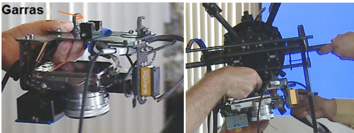
Figura E.8 Acomodo de las garras de la montura en el eje del dron
