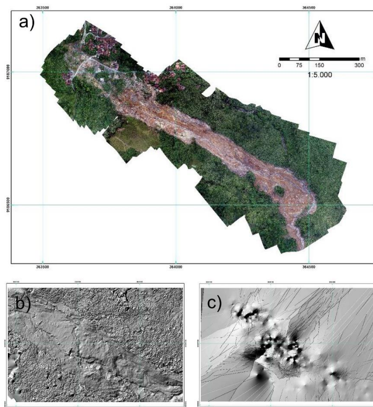
Figura 5.28 a) Ortofoto obtenida a partir de imágenes tomadas con un VANT, b) MDS obtenida por fotogrametría, c) MDE obtenido a partir de datos obtenidos con estación total y teodolito ( Permata et al. , 2016)
