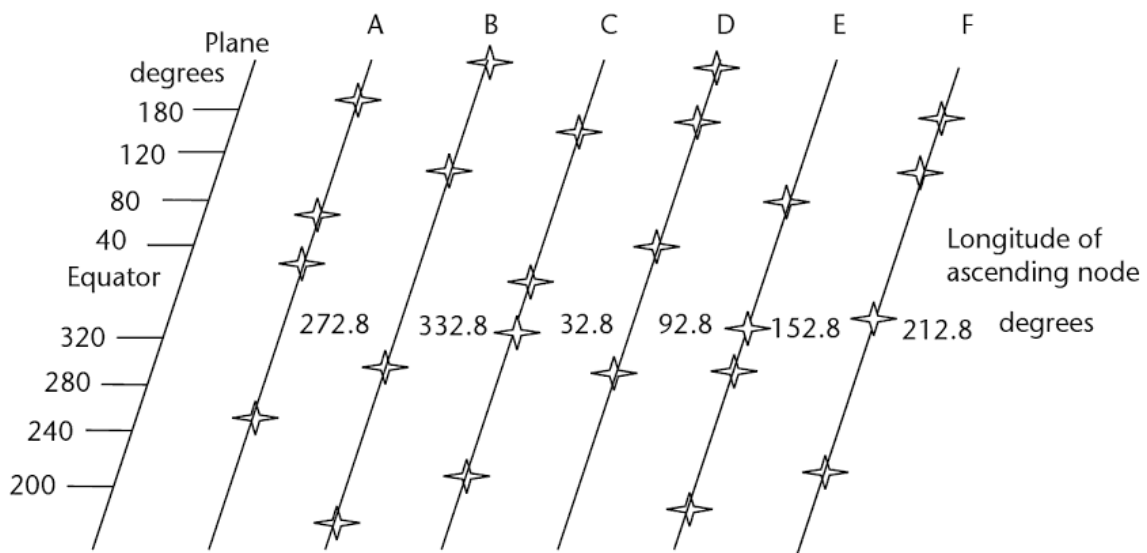
Figura 2.26 Proyección plana de la constelación GPS y sus órbitas (Kaplan y Hegarty, 2005)
